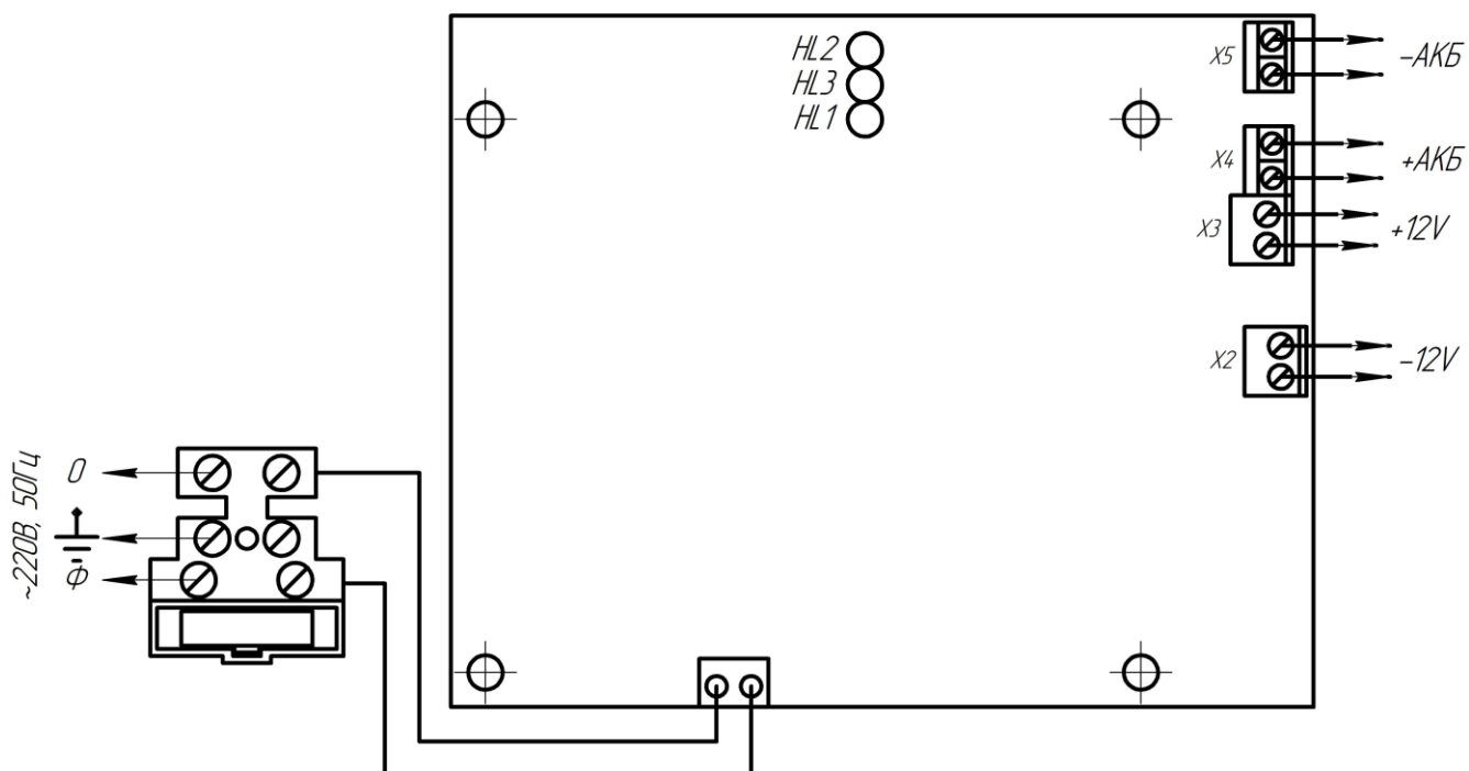
Рис. 1 Схема подключения
